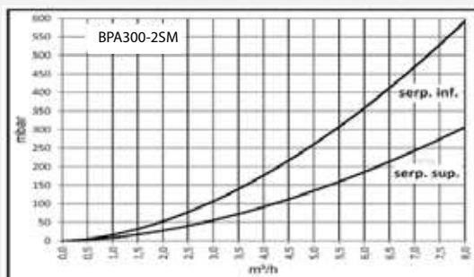
PERDITE DI CARICO SERPENTINE
