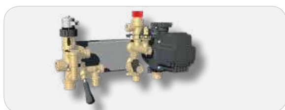
Gruppo idraulico compatto in ottone. Gruppo di mandata con deviatrice motorizzata, by-pass e rubinetto di carico impianto integrati. Circolatore ERP con sblocco pompa manuale su gruppo di ritorno.
